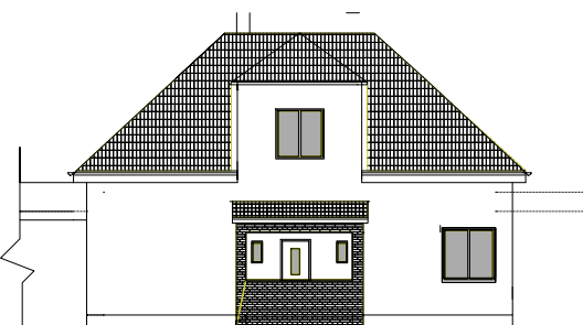
Pohled východní
