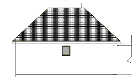
Pohled západní
